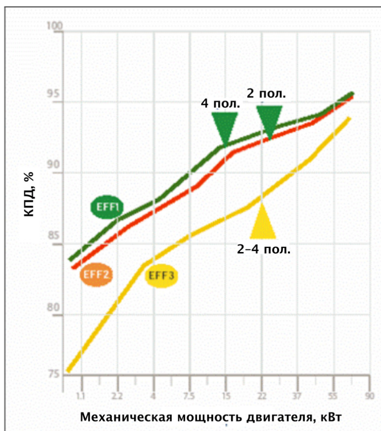
Рисунок 3.27: Энергоэффективность трехфазных индукционных электродвигателей
