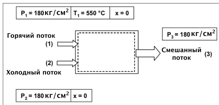
Рисунок 7.8. Смешивание двух потоков
