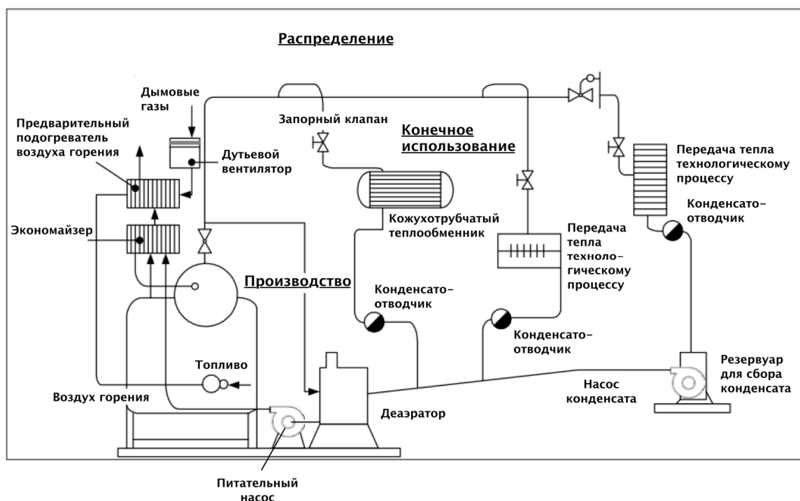
Рисунок 3.5: Типичная система производства и распределения пара [123, US_DOE]
