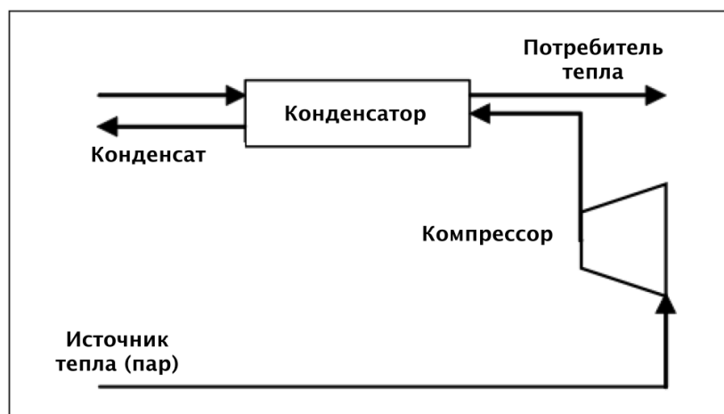
Рисунок 3.10: Схема процесса МРП
