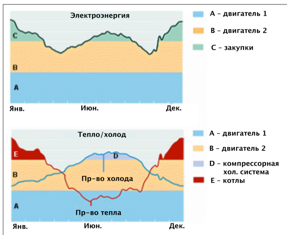
Рисунок 3.19: Оптимизация работы предприятия в течение года за счет тригенерации
