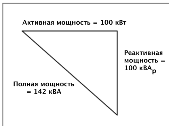
Рисунок 3.22: Активная, реактивная и полная мощность
