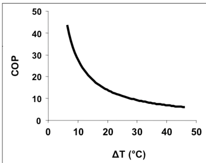
Рисунок 3.11: Коэффициент преобразования (COP) в зависимости от величины повышения температуры для типичного процесса МРП
