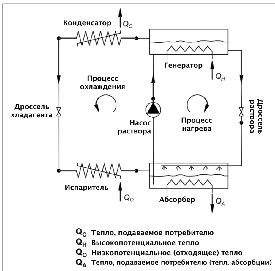
Рисунок 3.9: Схема абсорбционного теплового насоса
