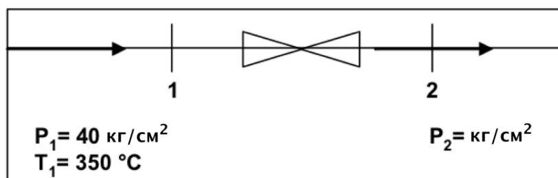
Рисунок 7.2. Процесс дросселирования пара
