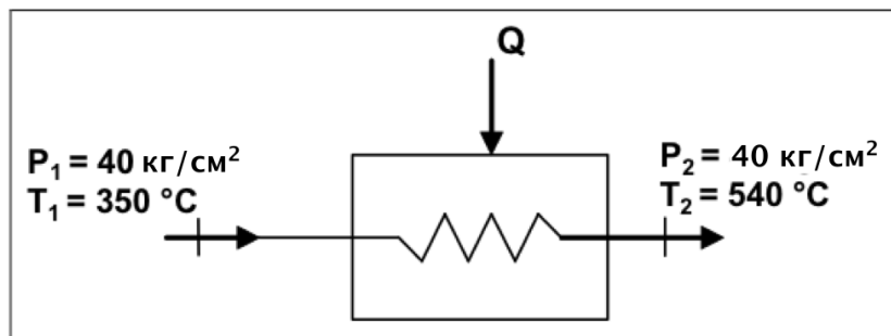
Рисунок 7.5: Нагрев пара в пароперегревателе
