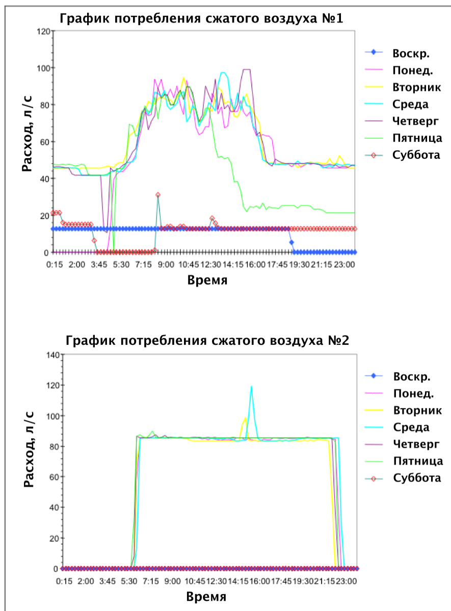
Рисунок 3.33: Графики потребностей в сжатом воздухе для двух систем [168, PNEUROP, 2007]
