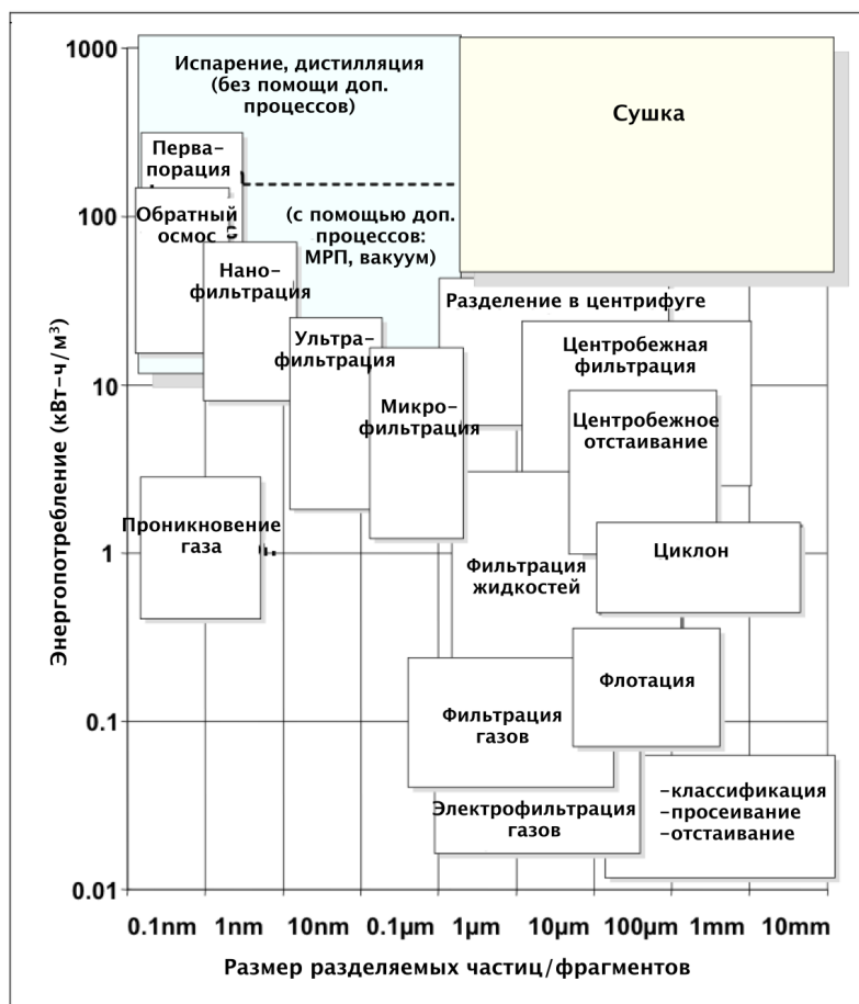
Рисунок 3.44: Энергопотребление некоторых процессов разделения [248, ADEME, 2007]
