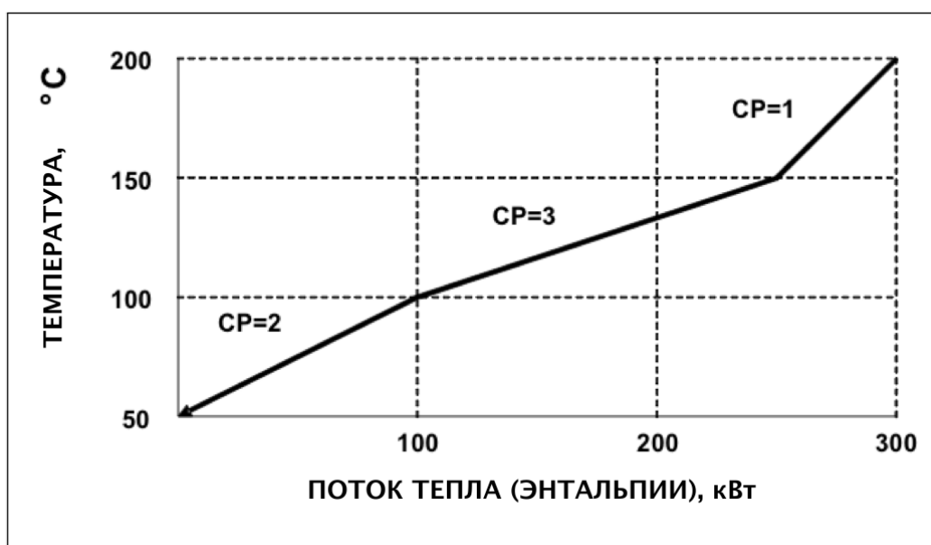
Рисунок 2.12. Горячая составная кривая
