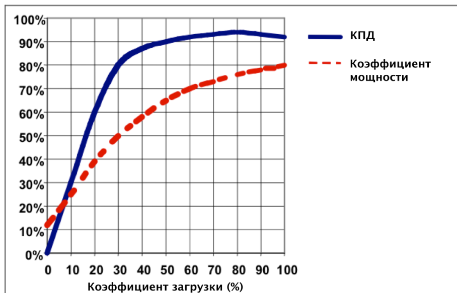
Рисунок 2.17: Зависимость коэффициента мощности устройства от коэффициента загрузки
