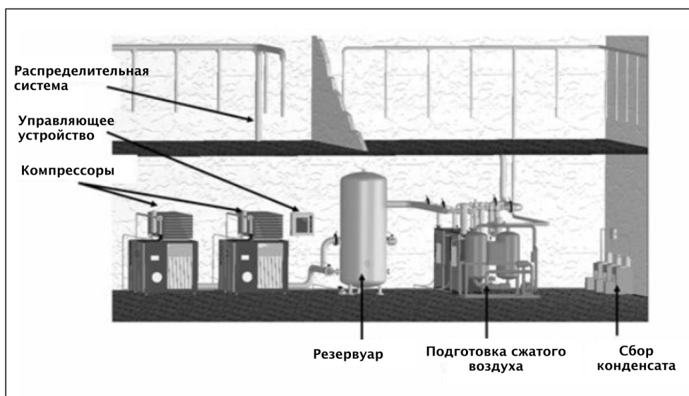
Рисунок 3.31: Типичные компоненты системы сжатого воздуха
