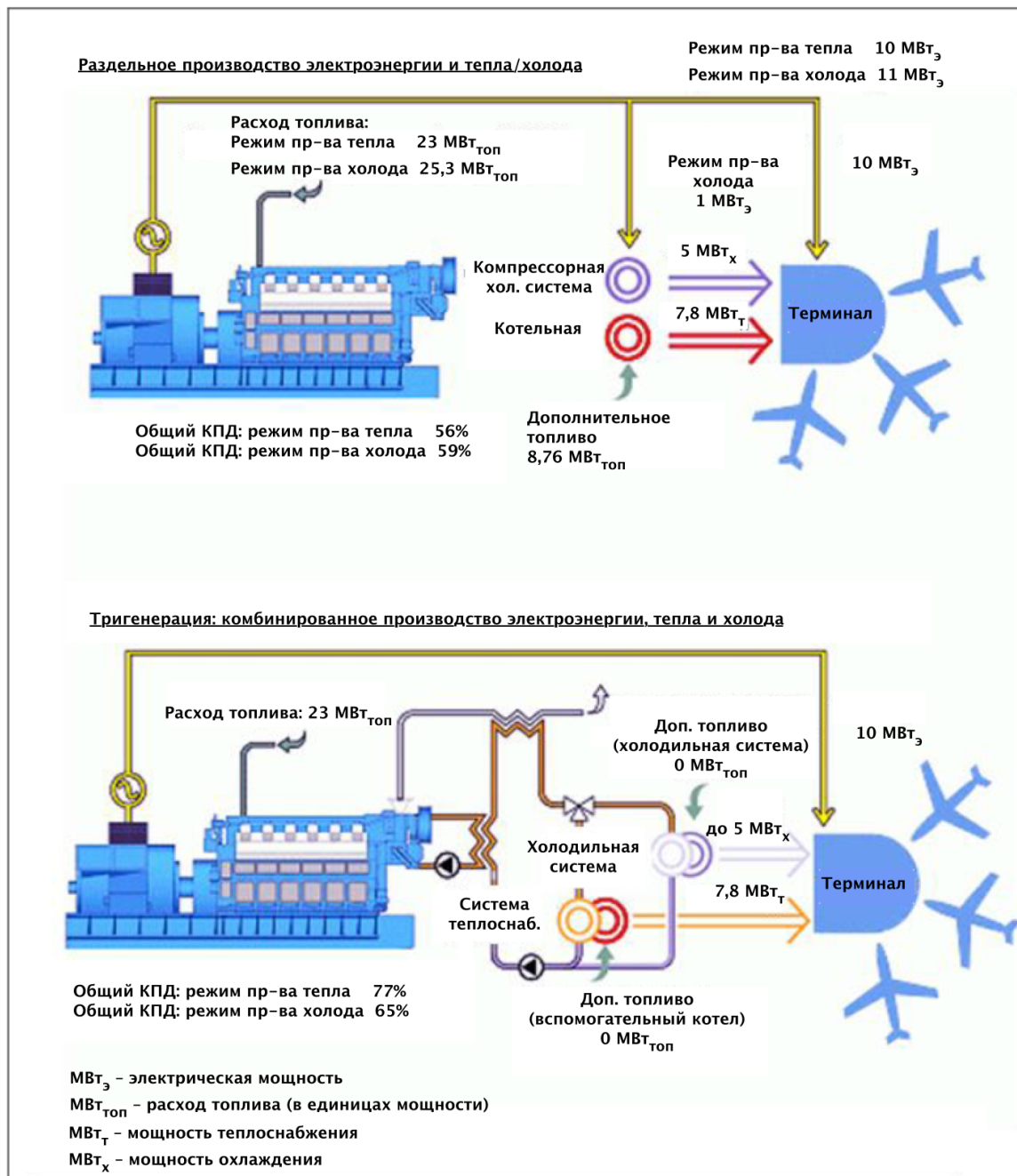
Рисунок 3.18: Сравнение тригенерации и раздельного производства энергетических продуктов для крупного аэропорта
