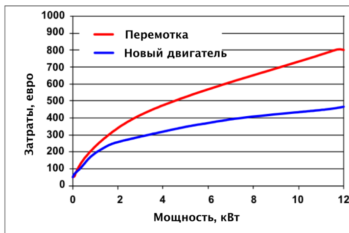
Рисунок 3.29: Затраты, связанные с приобретением нового двигателя и перемоткой существующего
