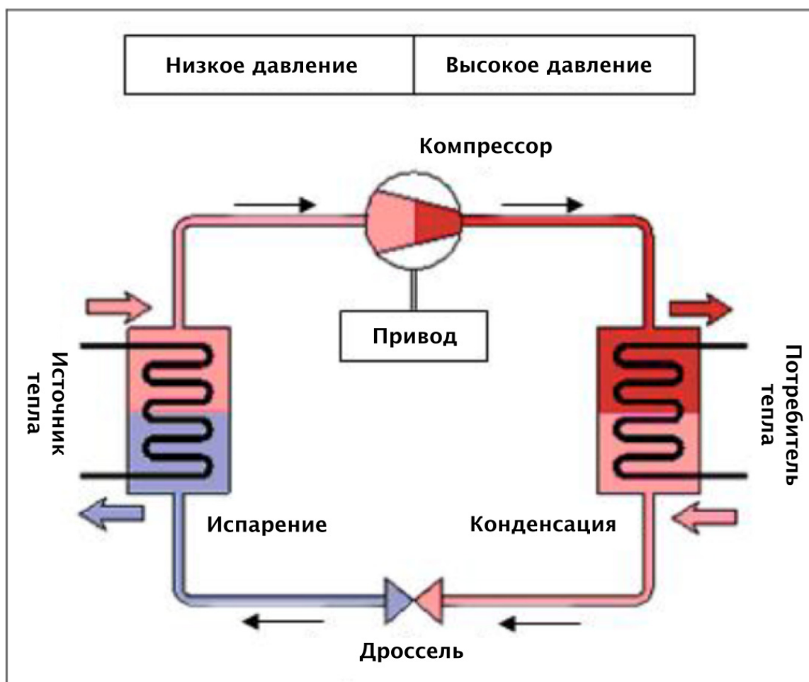
Рисунок 3.8: Схема компрессионного теплового насоса
