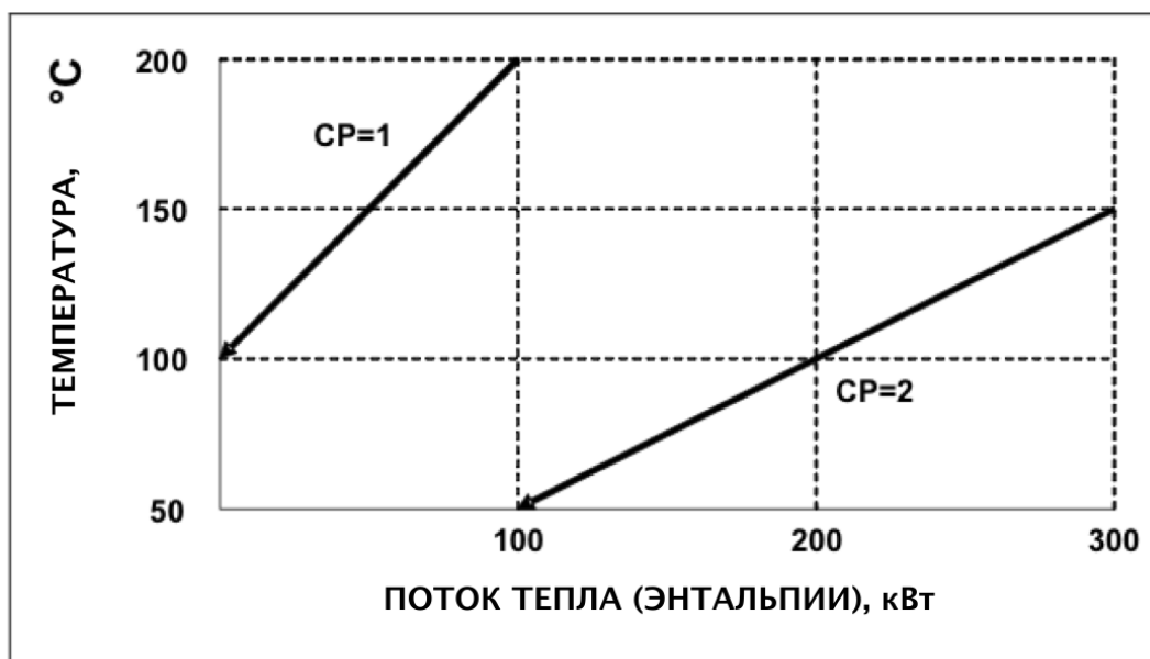
Рисунок 2.11: Два горячих потока
