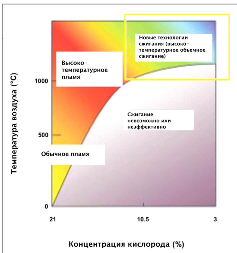
Рисунок 3.4: Различные режимы сжигания
