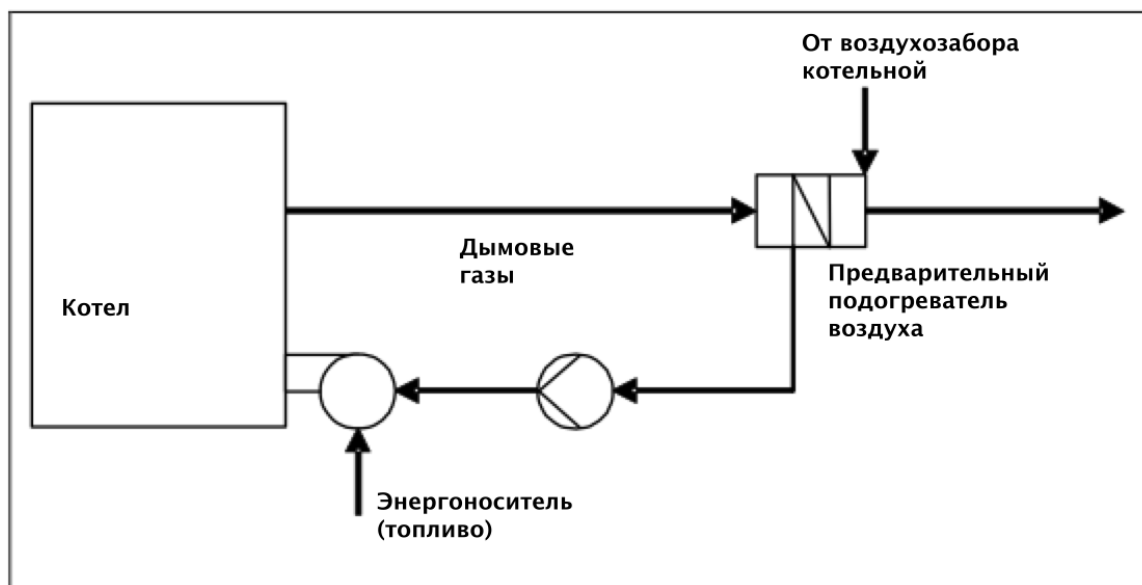
Рисунок 3.2.: Схема системы сжигания с предварительным подогревом воздуха
