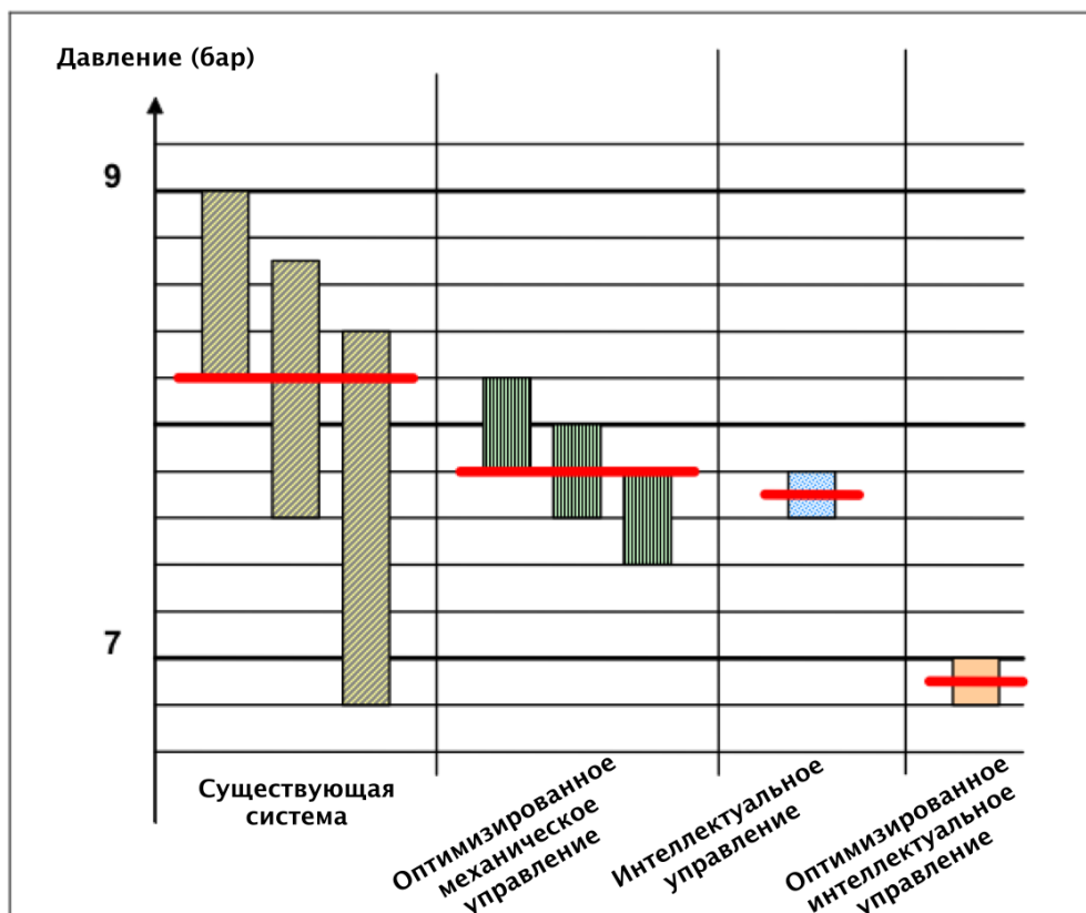
Рисунок 3.34: Различные подходы к управлению работой компрессора
