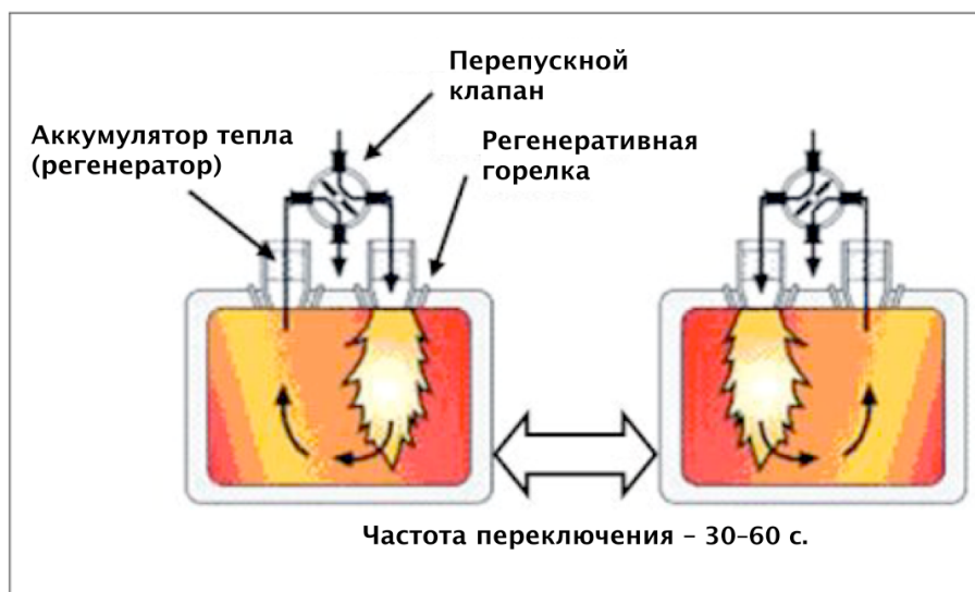
Рисунок 3.3. Принцип работы регенеративных горелок
