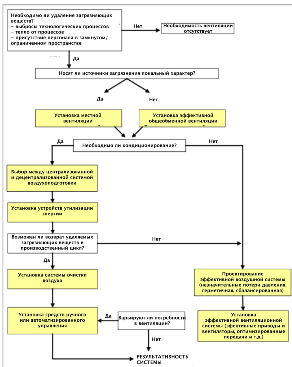
Рисунок 3.42: Блок-схема принятия решений по оптимизации энергопотребления вентиляционной системы
