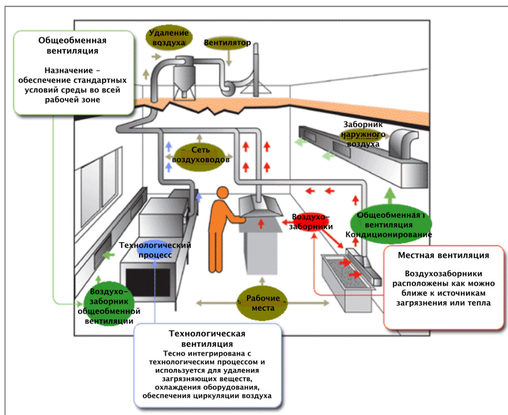
Рисунок 3.41: Вентиляционная система
