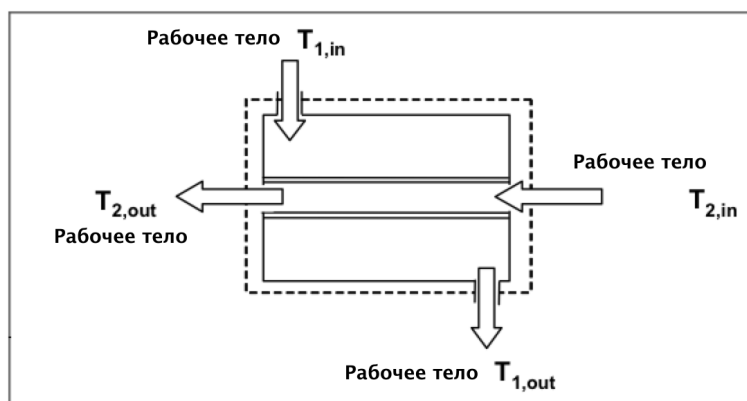
Рисунок 7.4: Противоточный теплообменник
