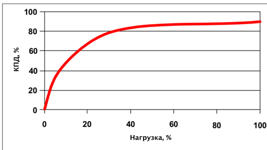
Рисунок 3.28: Зависимость КПД электродвигателя от его нагрузки
