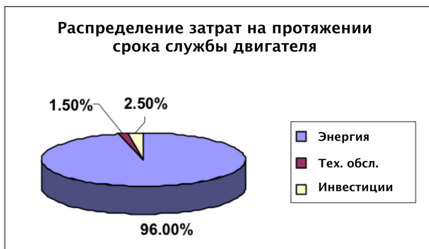
Рисунок 3.30: Затраты на протяжении срока службы электродвигателя
