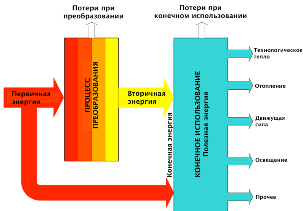
Рисунок 1.6: Определение первичной, вторичной и конечной энергии
