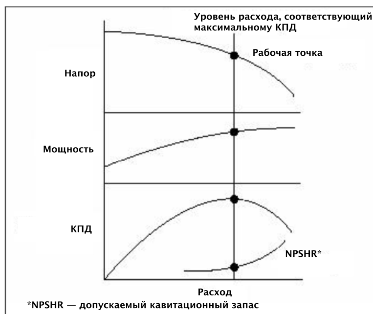
Рис. 3.35: Зависимость напора, мощности и КПД от расхода и точка максимального КПД [199, TWG]
